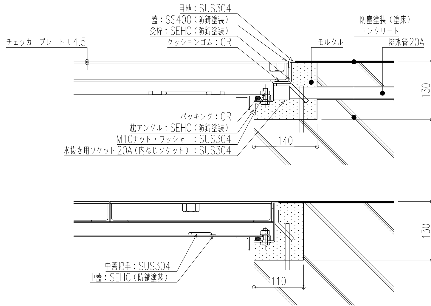
施工参考拡大図
